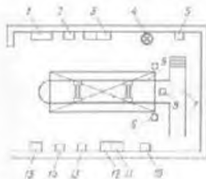
Рисунок 7.2. Схема универсального поста ТО-2.
