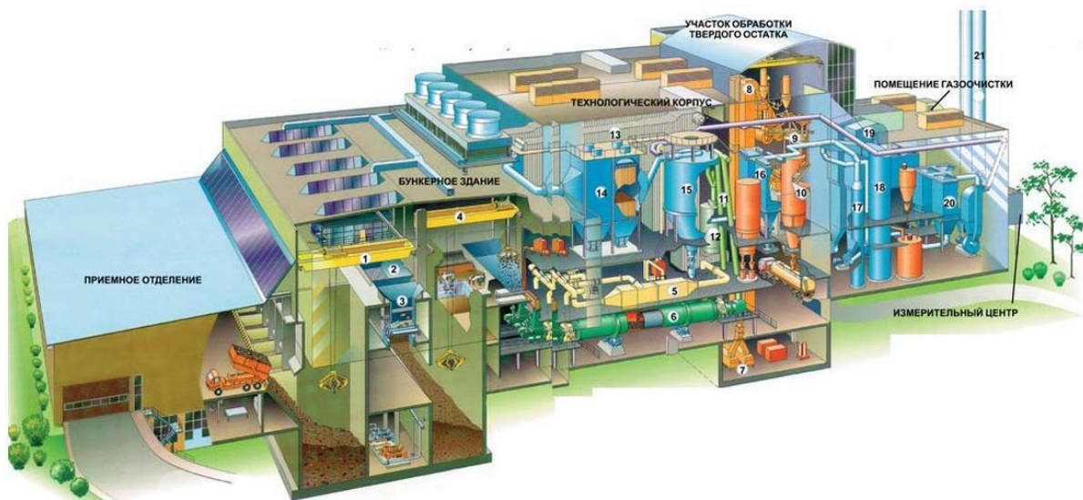
Рисунок 5.27. Технологическая схема мусороперерабатывающего завода.
