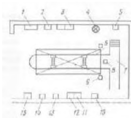
Рисунок 7.2. Схема универсального поста ТО-2.
